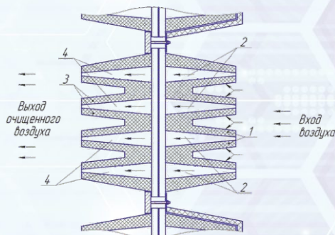
Схема 2-х ступенчатой очистки
