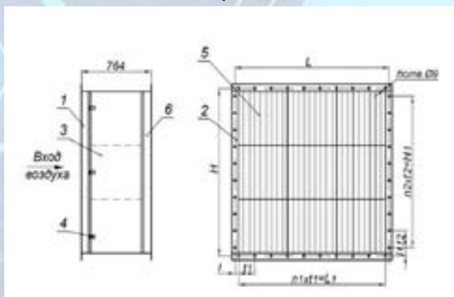
Рис.3 Схема секции компактных фильтров
