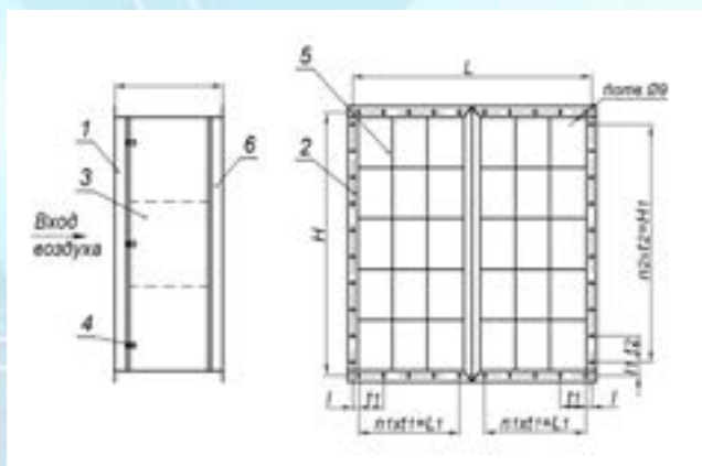
Рис.4 Схема секции компактного фильтра ССФ-К6 2/6x5; 2/6x6
