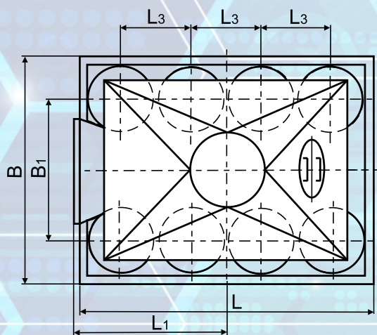
Рис.9 Циклон типа ЦН-15х4СП
