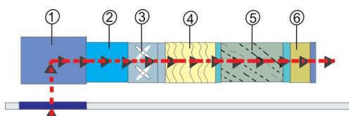
Рис.1 Схема фильтрации
