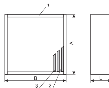
Рис.1 Схема фильтра ФяС-Ф.
